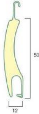
LAMA ALUMIVENT
