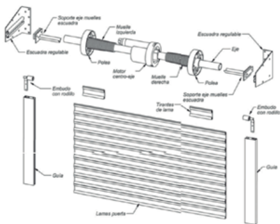
DESGLOSE DE PIEZAS
