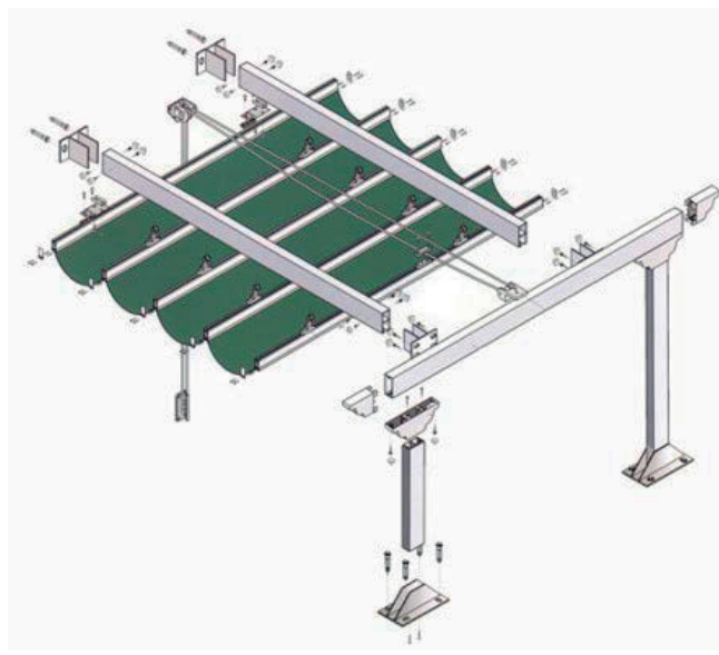
MONTAJE A TECHO
