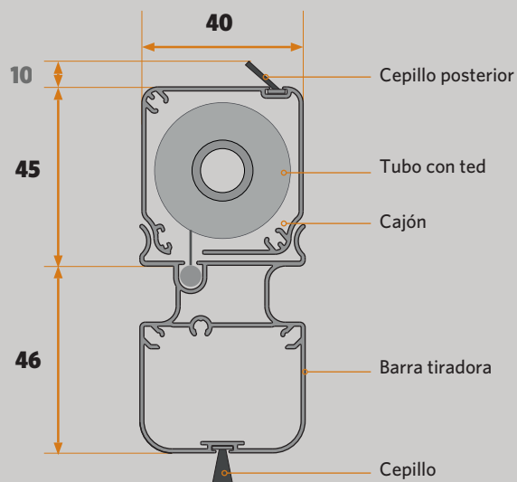
Sección horizontal
