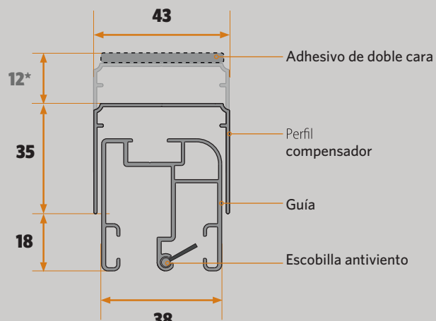
Sección vertical
