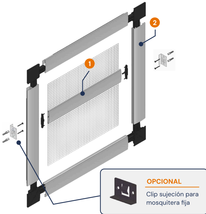
PERFIL TRAVESAÑO
